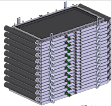
Flowrox Paquete de placas TP 32 16 2 45 C
