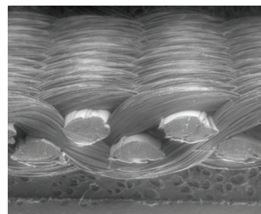
Фильтроткань Flowrox W-TA220L; изображение, полученное с помощью электронного микроскопа
