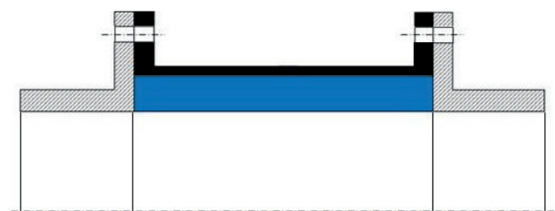
Единственная часть вставки, контактирующая с рабочей средой, это стойкое к абразивному истиранию полиуретановое покрытие.
